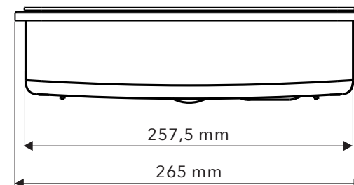
Pohľad predný
